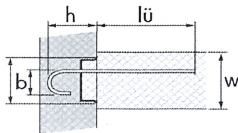
Bügel-Typen RB4 zweischneittig
