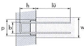
Bügel-Typen RB4 zweischneittig
