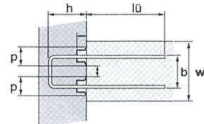
Konsol-Typen RB5 zweischneittig
