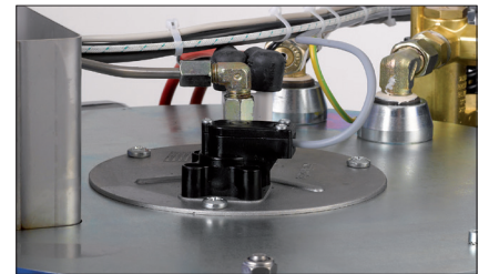
Optische Flammüberwachung
