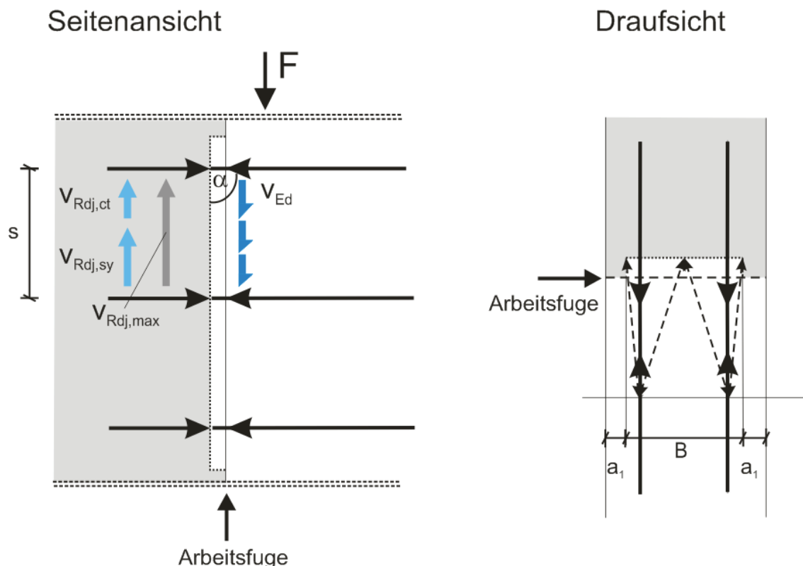
Abbildung 3: Stabwerkmodell zur Querkräfteübertragung in Betonierfugen für den Fall a des DBV-Merkblatt /2/ für a_1 < 5\text{cm}
