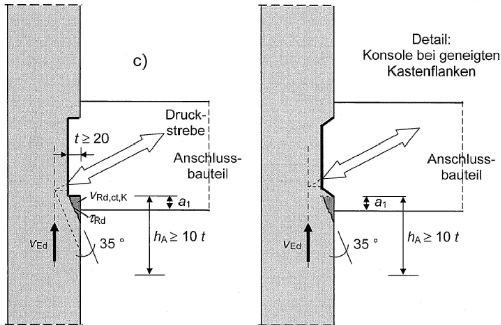
Abbildung 6: vereinfachtes Tragmodell des Konsolentrageanteils nach /3/, Bild 9
