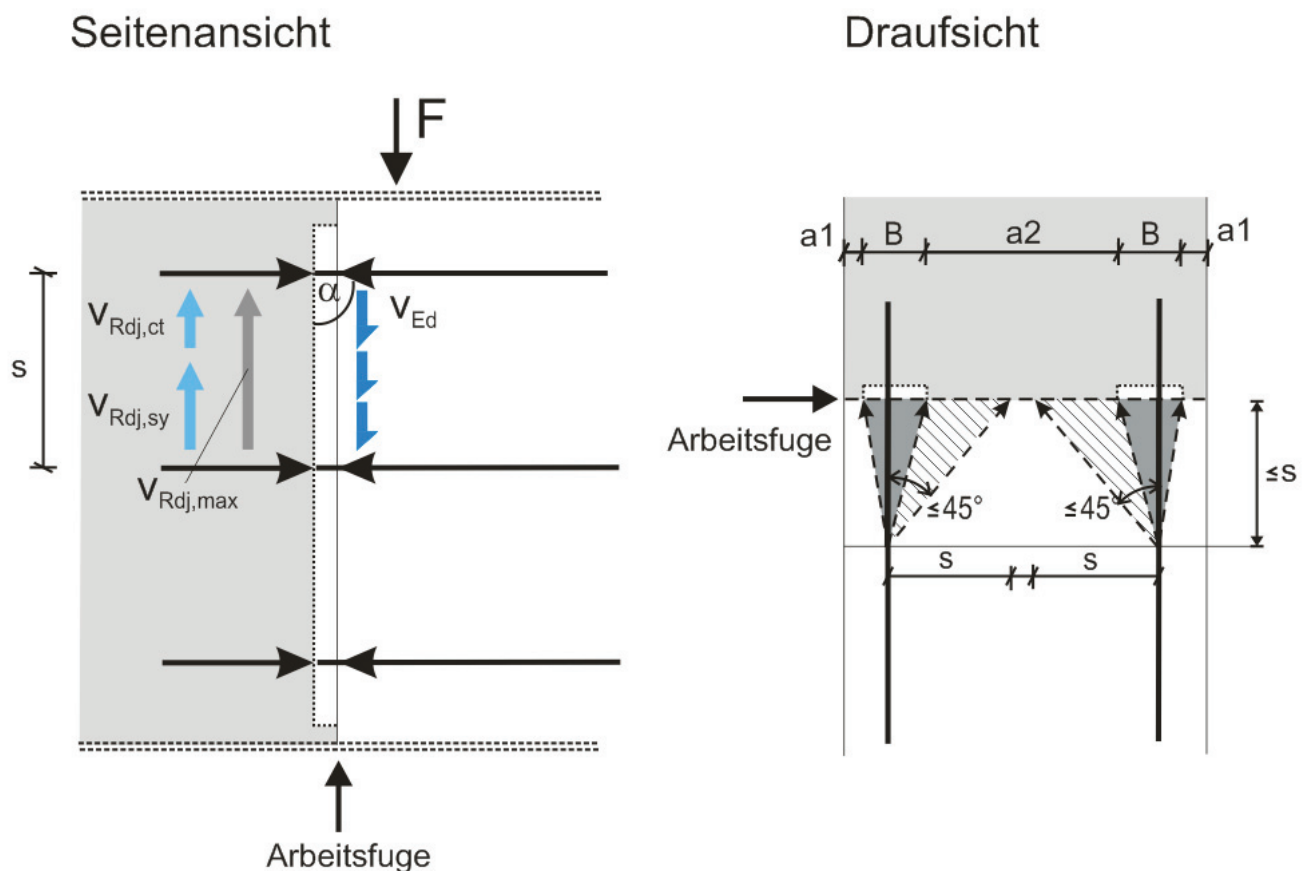
Abbildung 4: Stabwerkmodell zur Querkräfteübertragung in Betonierfugen für den Fall b nach DBV-Merkblatt /2/ für a_1 < 5 \text{ cm} und a_2 \geq 5 \text{ cm}
