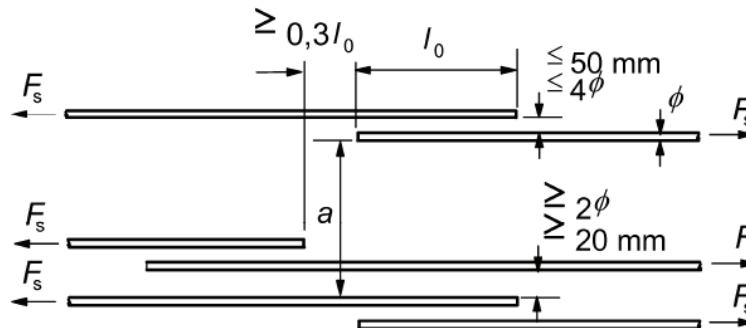
Abbildung 2 Anordnung gestoßener Stäbe nach EC 2, Bild 8.7
