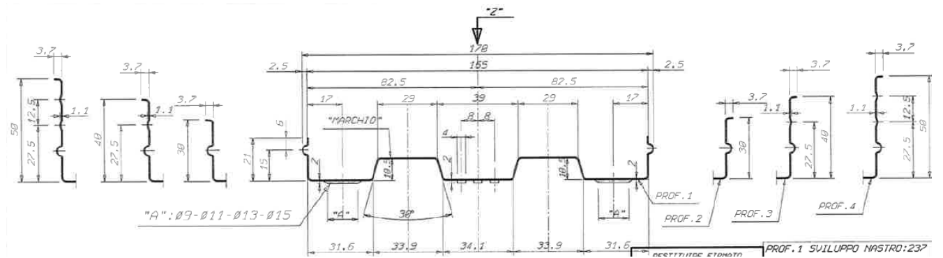
Abbildung 7 Geometrie Rübox QW/165 – querverzahnter Verwahrkasten für \varnothing = 8, 10 und 12 mm
