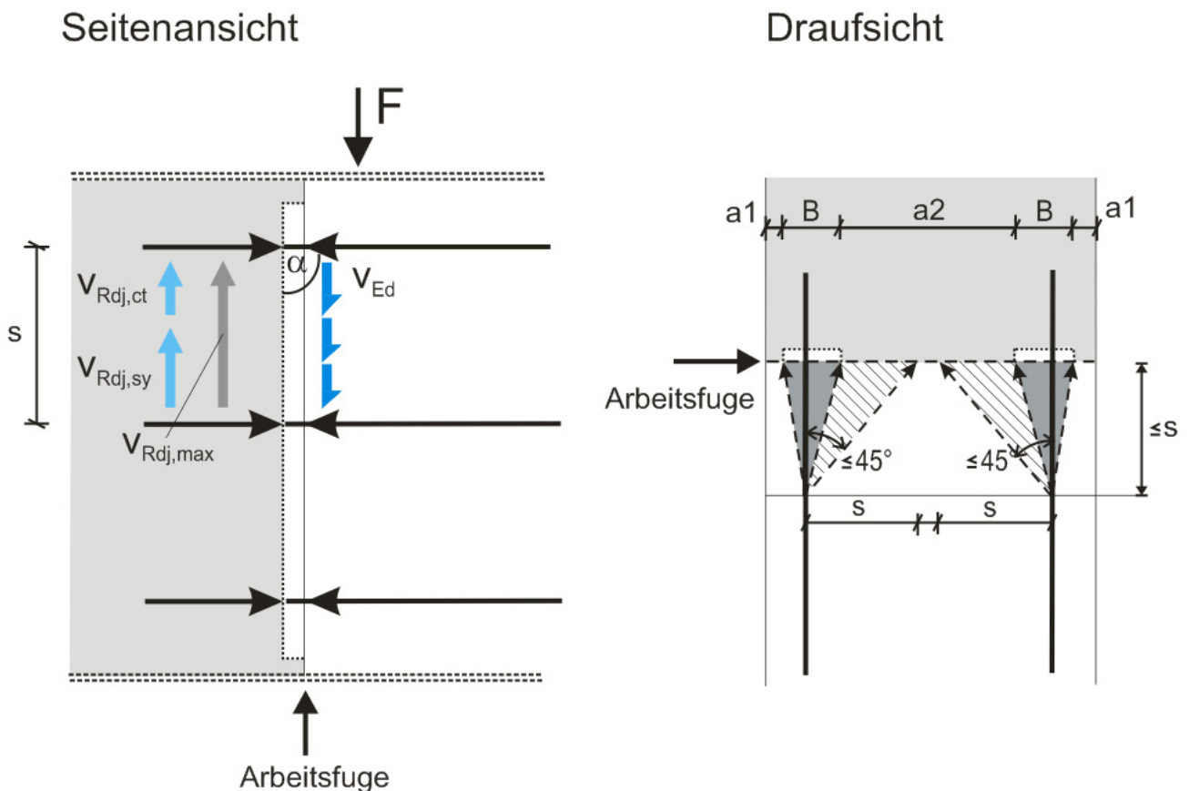
Abbildung 12: Stabwerkmodell zur Querkräfteübertragung in Betonierfugen für den Fall b nach DBV-Merkblatt /3/ für a 1 < 5 cm und a 2 ≥ 5 cm
