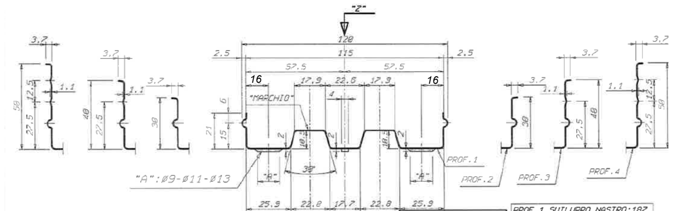
Abbildung 8 Geometrie Rübox QW/115 – querverzahnter Verwahrkasten für \varnothing = 8, 10 und 12 mm
