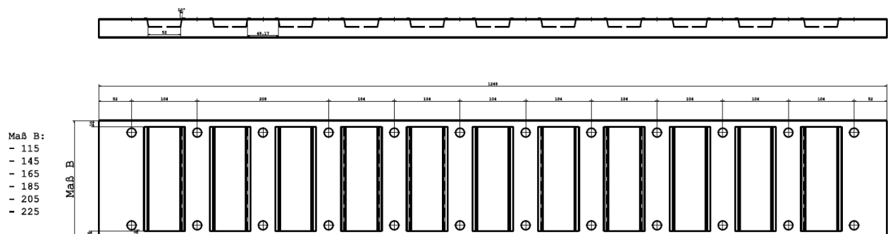
Abbildung 3 Geometrie Rübox QSI – längsverzahnter Verwahrkasten für Stababstand s = 10 cm
