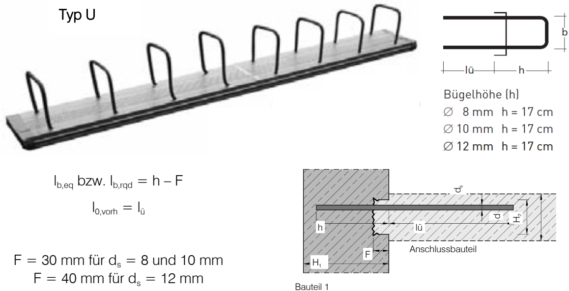
Abbildung 9: Definition der verankerten Stablängen des RÜBOX-Anschlusses mit den Bezeichnungen des RÜBOX-Kataloges
