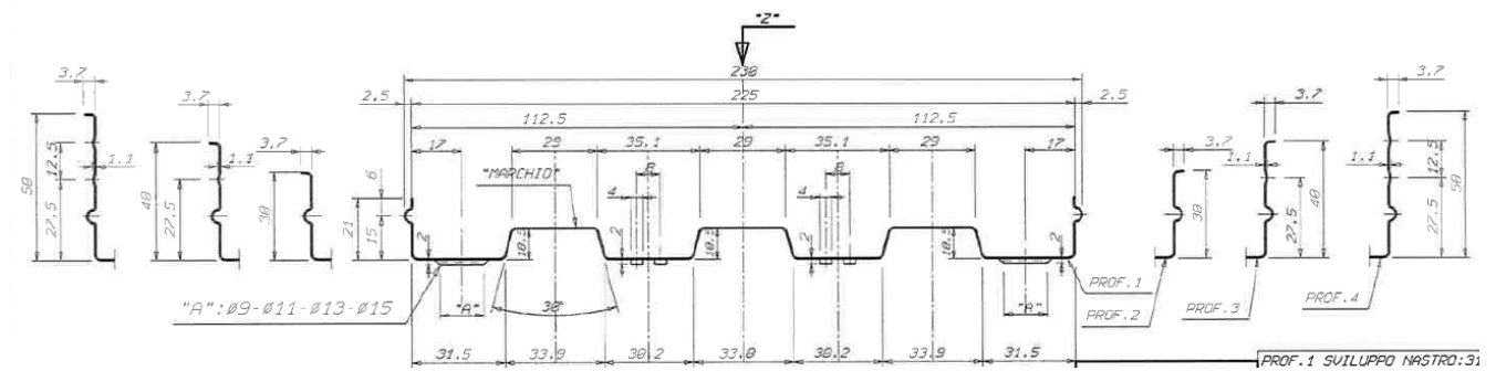
Abbildung 6 Geometrie Rübox QW/225 – querverzahnter Verwahrkasten für \varnothing = 8, 10 und 12 mm
