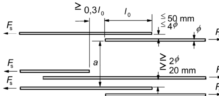
Abbildung 10 Anordnung gestoßener Stäbe nach EC 2, Bild 8.7
