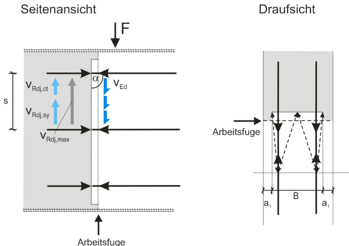
Abbildung 11: Stabwerkmodell zur Querkräfteübertragung in Betonierfugen für den Fall a des DBV-Merkblatt /2/ für a_1 < 5\text{cm}
